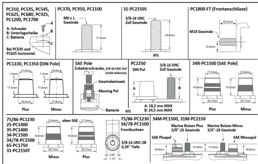
Abbildung 1: Maße der Pole und Anschlüsse
