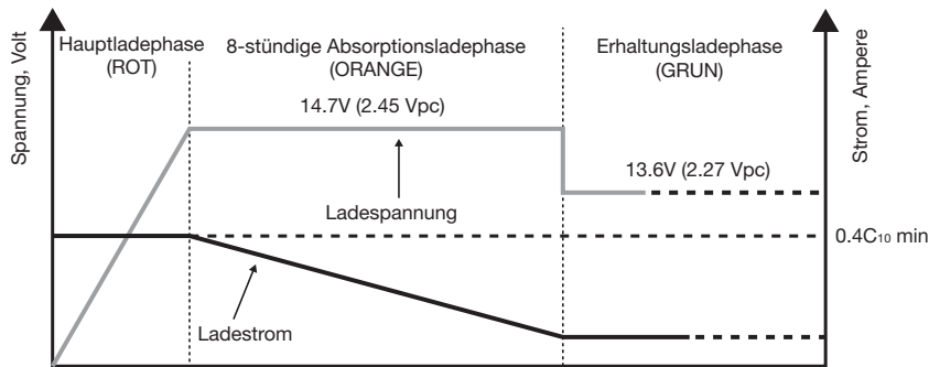
Abbildung 4: Empfohlenes 3-stufiges Ladeprofil für ODYSSEY® Batterien
