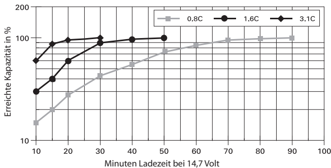
Abbildung 6: Ladezustände in Abhängigkeit von Ladestrom und Ladezeit
