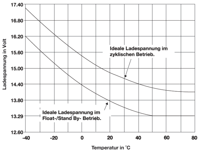
Abbildung 5: Ladespannung in Abhängigkeit der Umgebungstemperatur
