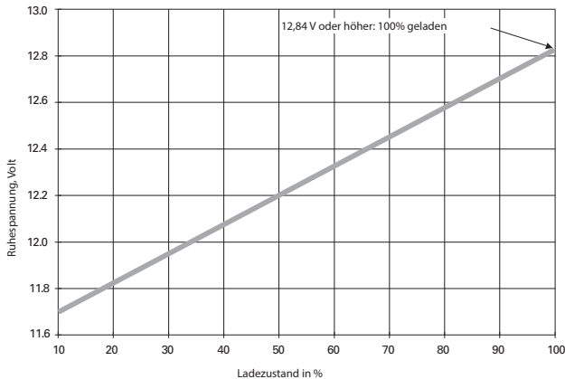
Abbildung 2: Ladezustand im Verhältnis zur Ruhespannung der ODYSSEY® Batterie
