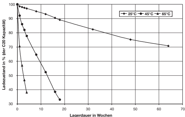
Abbildung 3: Lagerdauer für ODYSSEY® Batterien bei Umgebungstemperaturen von 25°C, 45°C, 65°C
